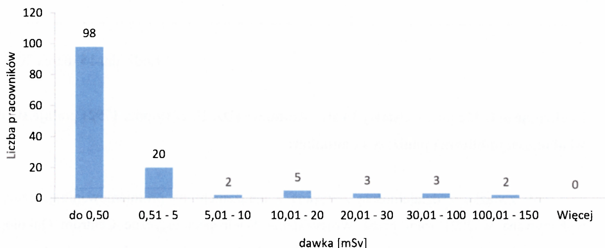
Wykres 2. Rozkład dawek na dłonie otrzymanych przez pracowników kategorii A i B w 2021 roku
